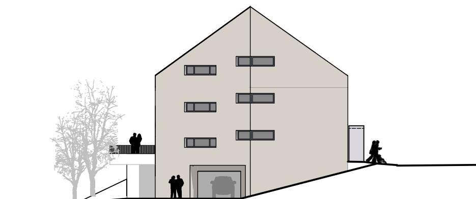
Ansicht Nord
